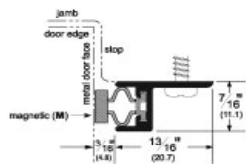
אטם משקוף מגנטי לדלת M_2815
