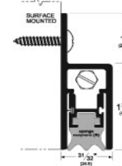
סף תחתון Pemko 430 RL
