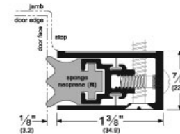
סף תחתון Pemko 430 RL
