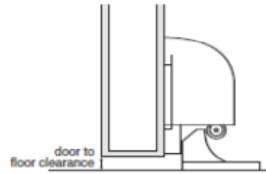
מעצור רצפה עם תפיסה עם תפיסה ROCKWOOD 491
