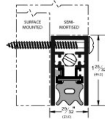
סף תחתון Pemko 4301 RL
