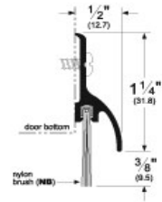
אף מיים מעל לדלת NB 3452
