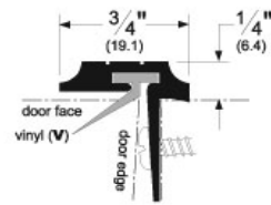
אטם בין כפיים ASTRAGAL
