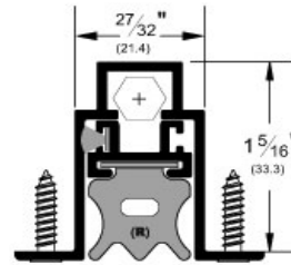
סף תחתון Pemko 434 RL
