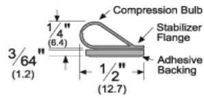
אטם משקוף לדלת S 88
