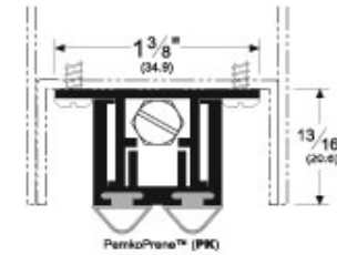
סף תחתון לדלתות אלומיניום Pemko 420
