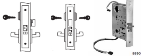
מנעול חבוי סדרה 800 פונקציות בהתאם לדרישות התפעוליות של הדלת כולל בהלה
